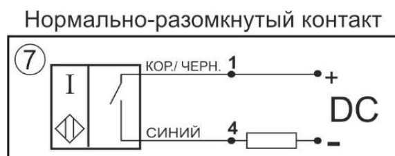
Схема соединения
