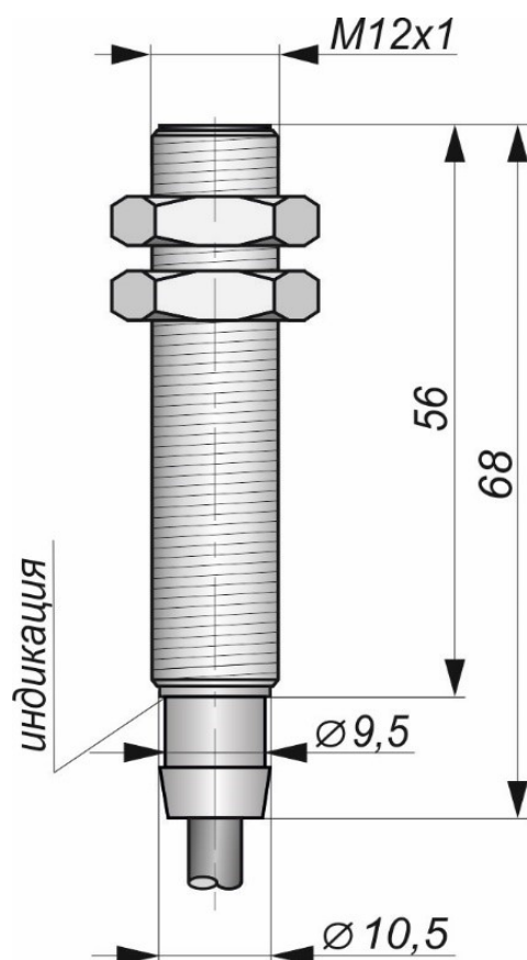
Габаритный чертеж
