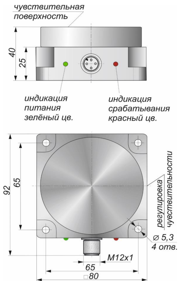
Габаритный чертеж
