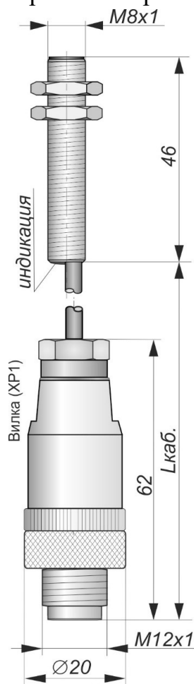
Габаритный чертеж
