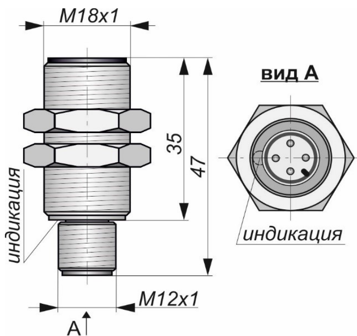
Габаритный чертеж
