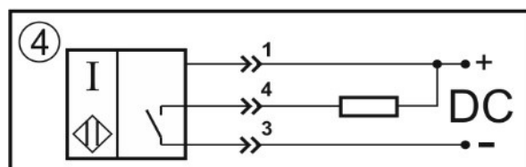
Нормально-разомкнутый контакт
