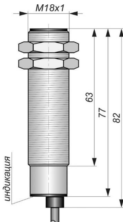
Габаритный чертеж
