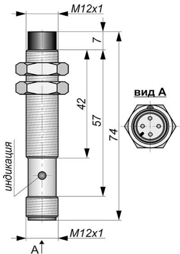
Габаритный чертеж
