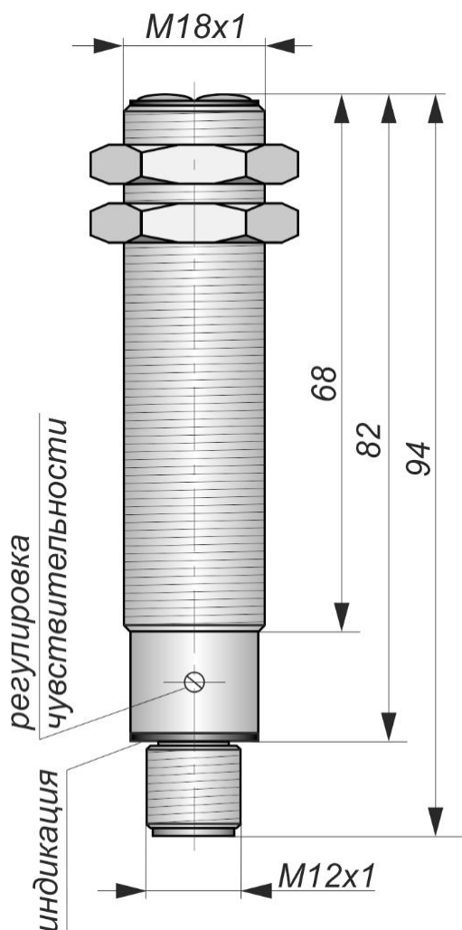
Габаритный чертеж
