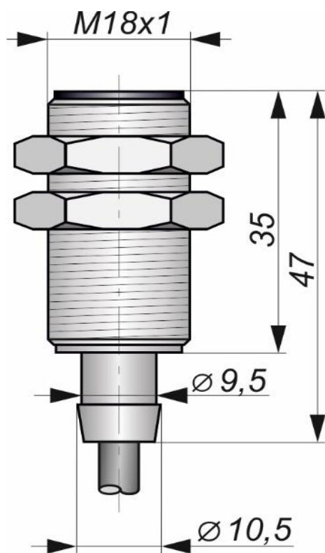
Габаритный чертеж
