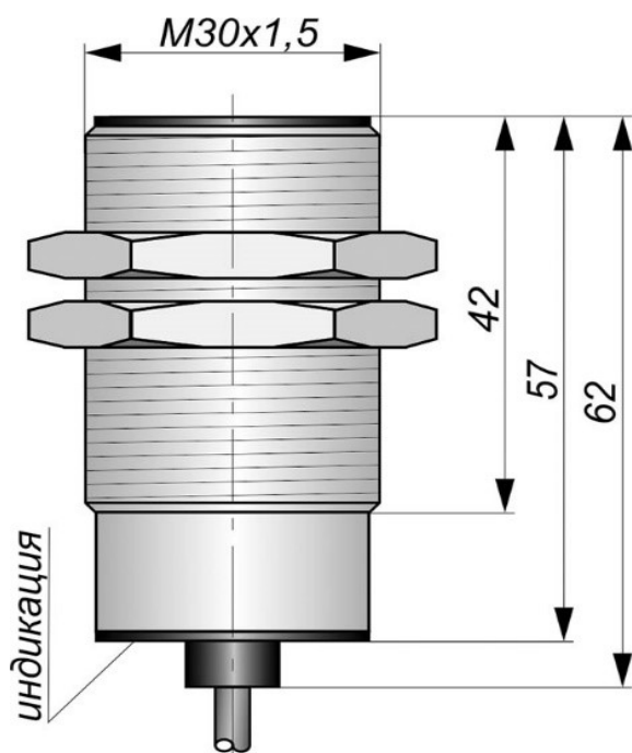
Габаритный чертеж
