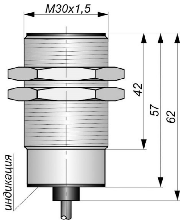
Габаритный чертеж
