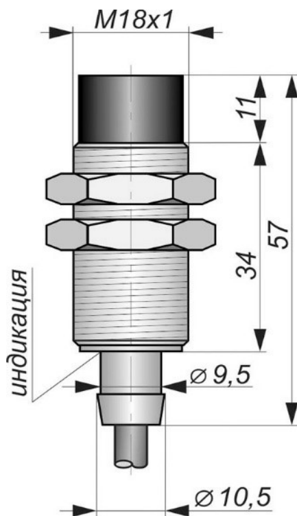
Габаритный чертеж
