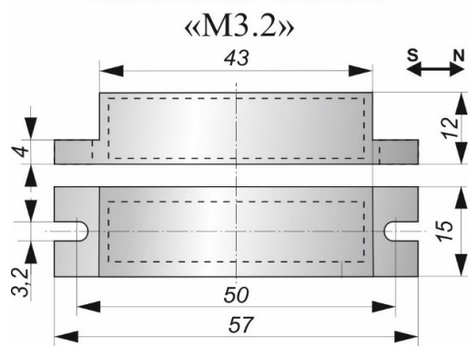
Магнитная система
