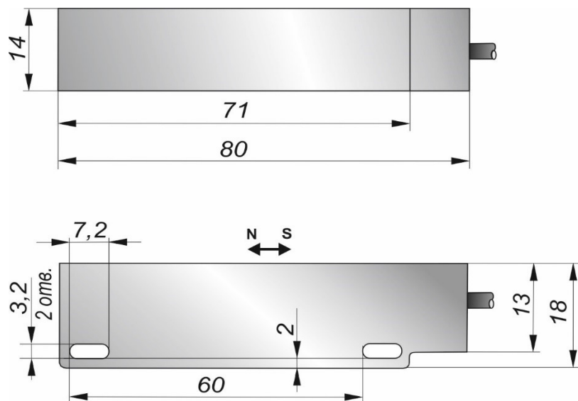
Габаритный чертеж
