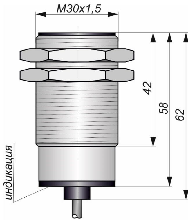
Габаритный чертеж
