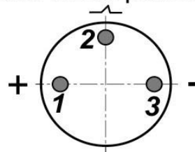
Цоколевка разъема
