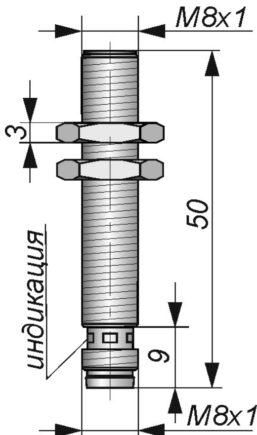
Габаритный чертеж
