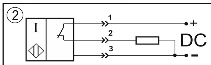
Нормально-замкнутый контакт
