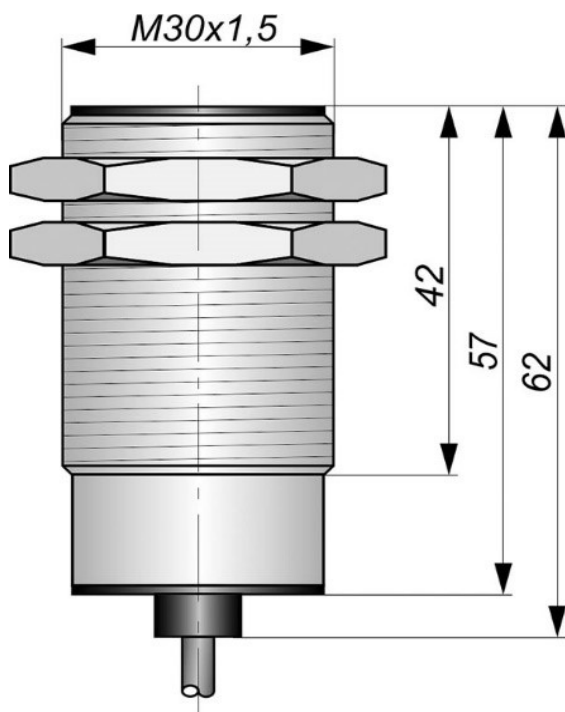
Габаритный чертеж
