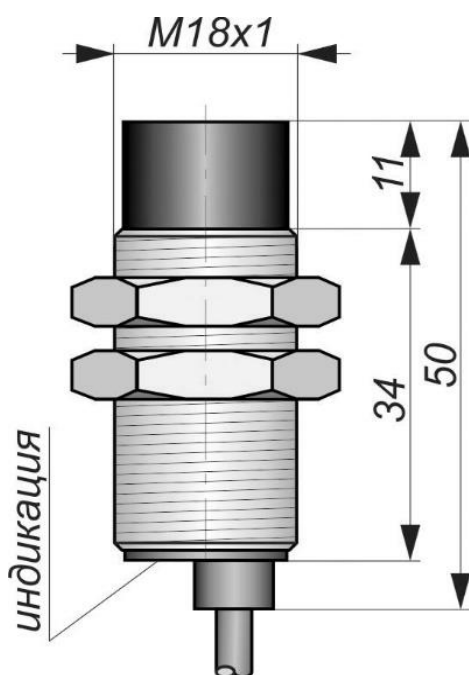
Габаритный чертеж
