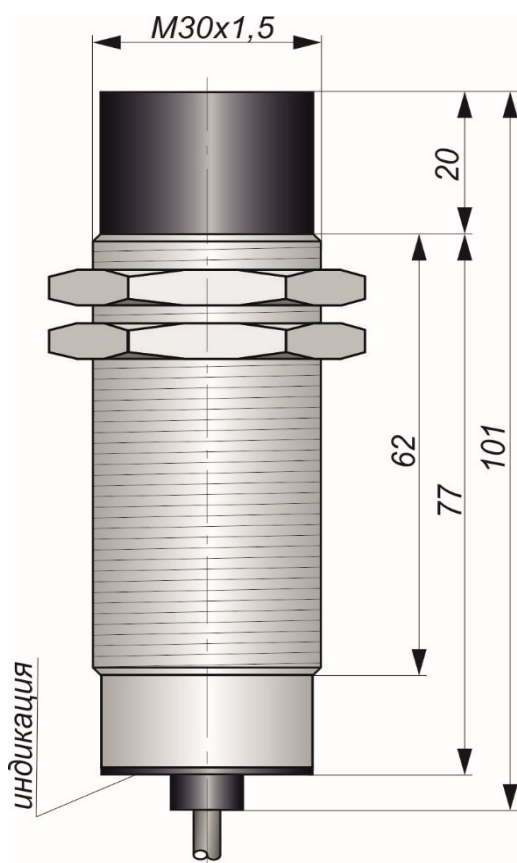
Габаритный чертеж
