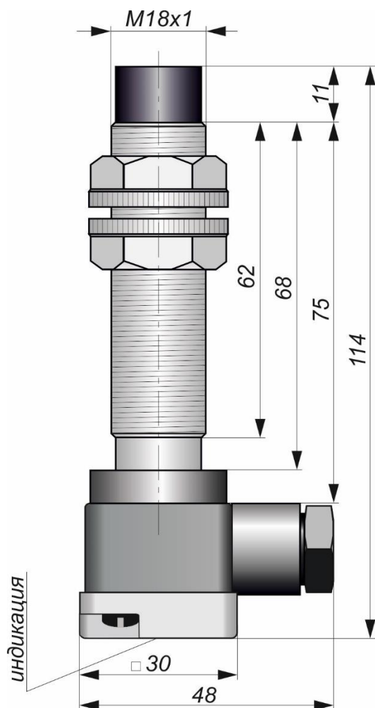
Габаритный чертеж
