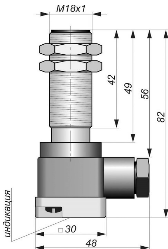
Габаритный чертеж
