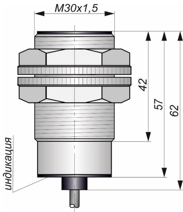
Габаритный чертеж
