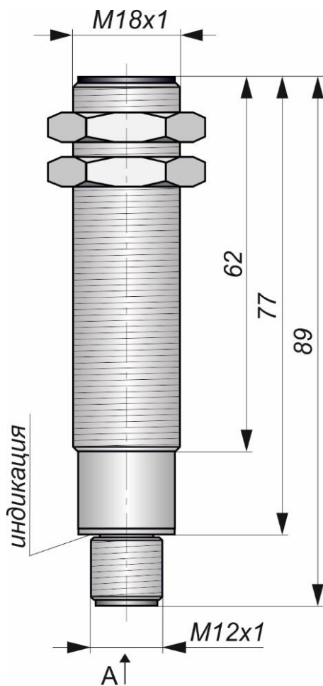
Габаритный чертеж
