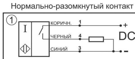
Схема соединения
