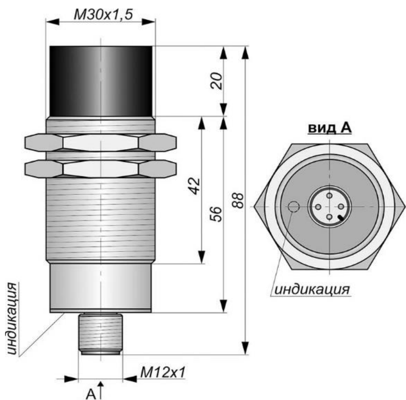
Габаритный чертеж
