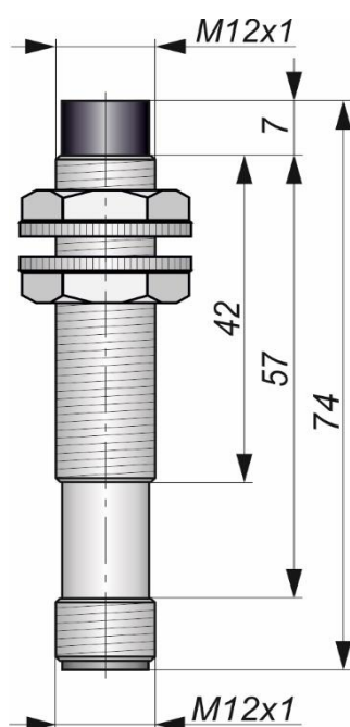
Габаритный чертеж
