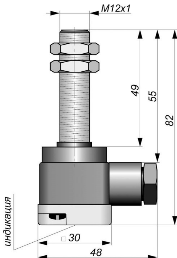
Габаритный чертеж
