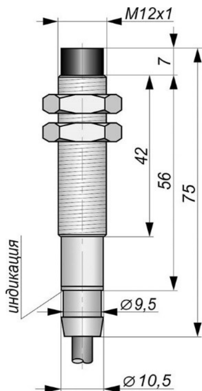
Габаритный чертеж
