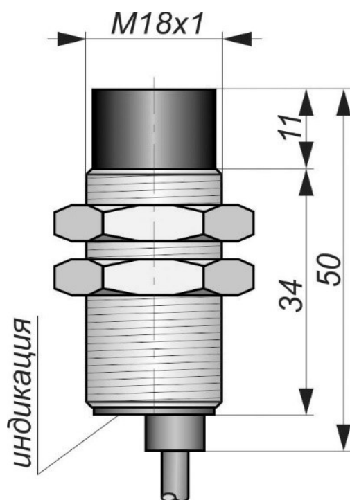
Габаритный чертеж
