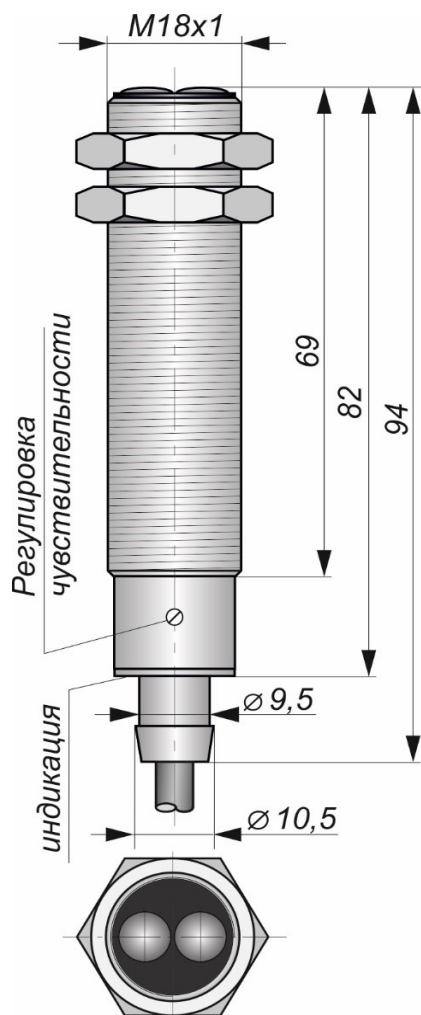
Габаритный чертеж
