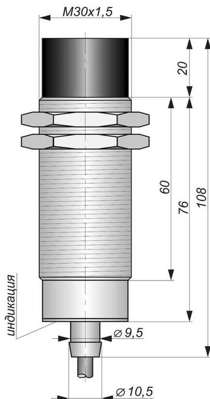
Габаритный чертеж
