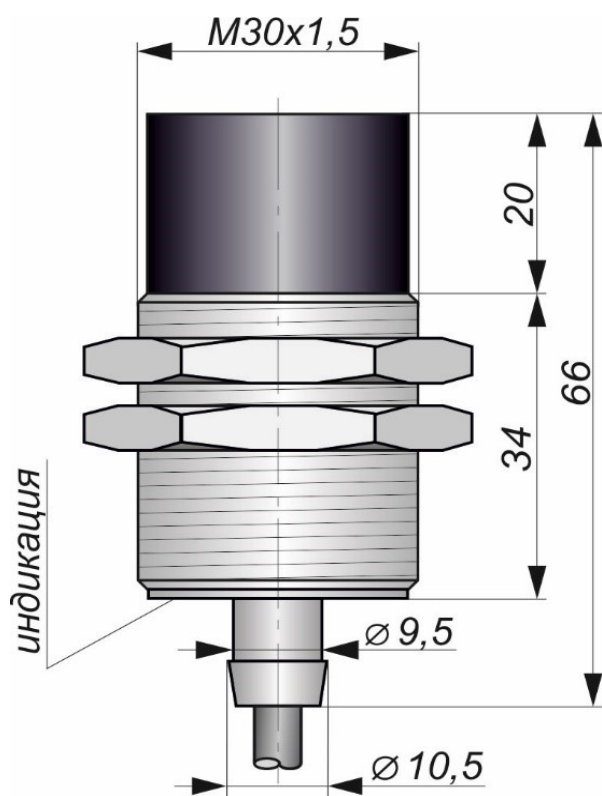
Габаритный чертеж
