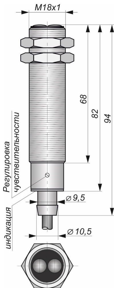
Габаритный чертеж
