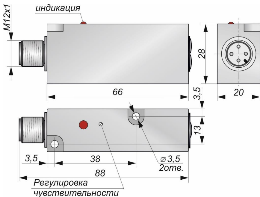
Габаритный чертеж
