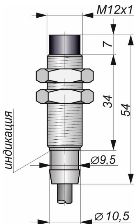
Габаритный чертеж
