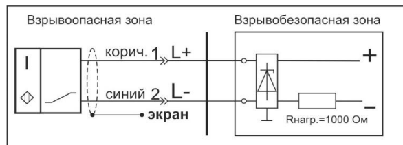
Схема соединения
