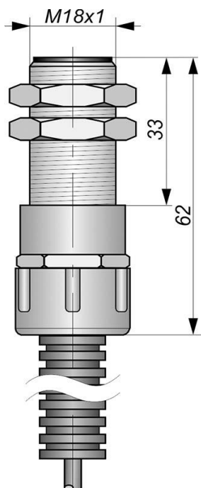
Габаритный чертеж
