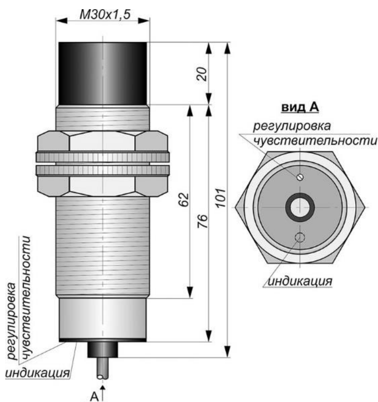
Габаритный чертеж
