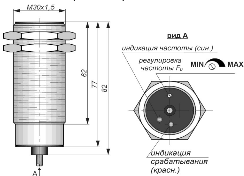
Габаритный чертеж
