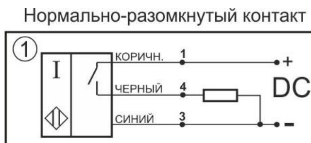
Схема соединения
