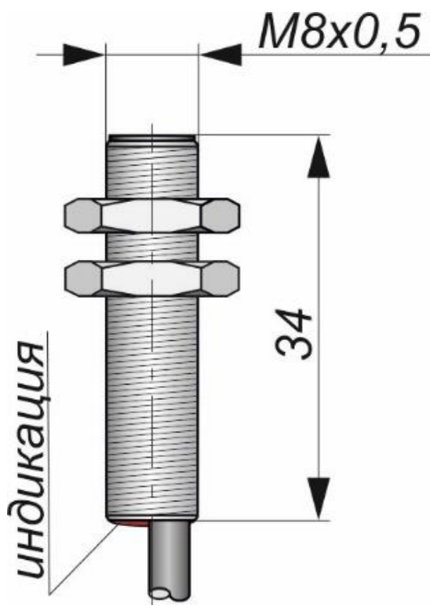
Габаритный чертеж
