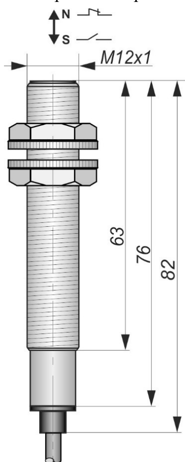
Габаритный чертеж
