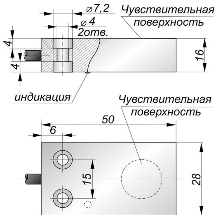
Габаритный чертеж
