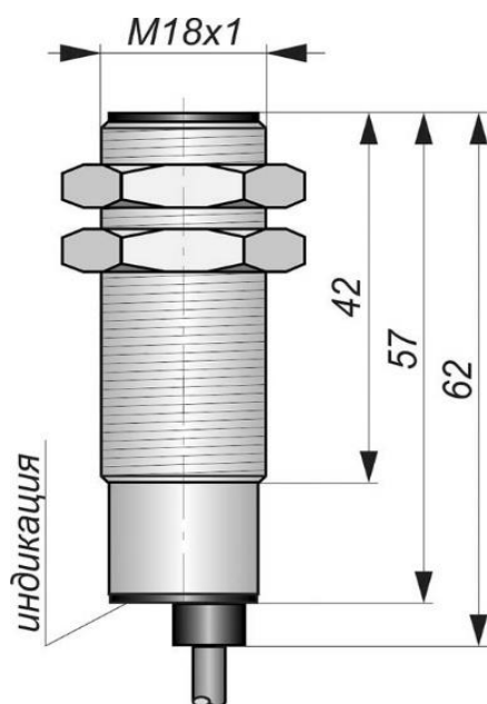
Габаритный чертеж
