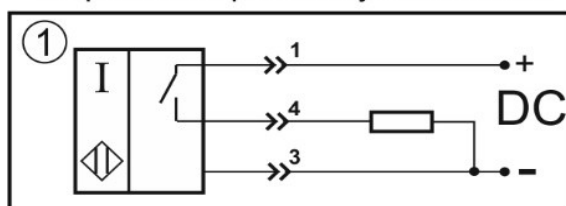
Нормально-разомкнутый контакт
