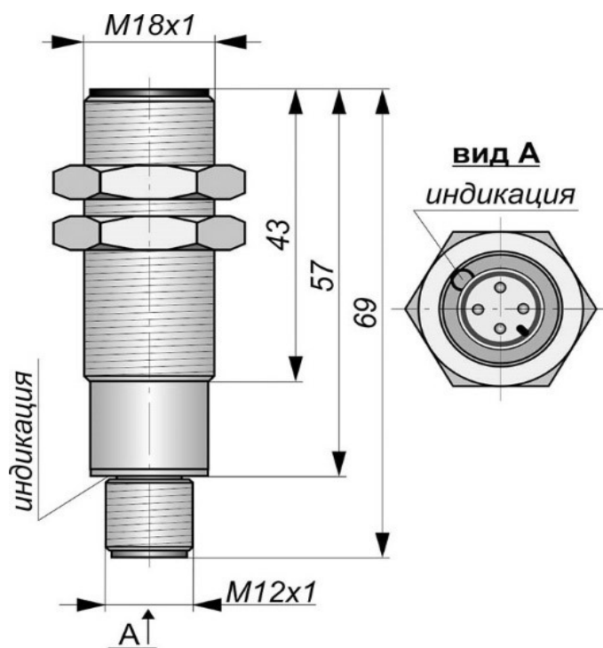
Габаритный чертеж
