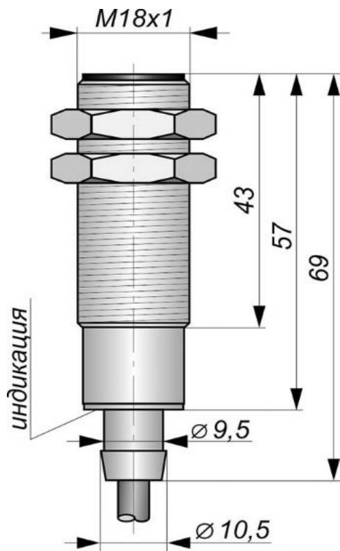
Габаритный чертеж
