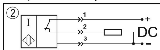
Нормально-замкнутый контакт
