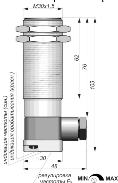
Габаритный чертеж
