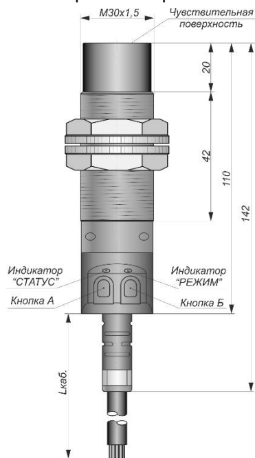
Габаритный чертеж
