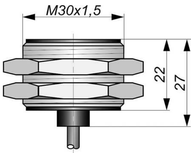
Габаритный чертеж
