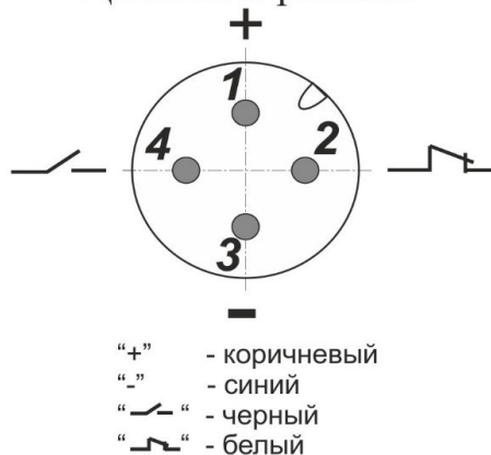
Цоколевка разъема
