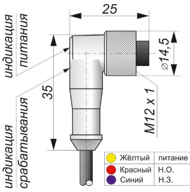
Габаритный чертеж
