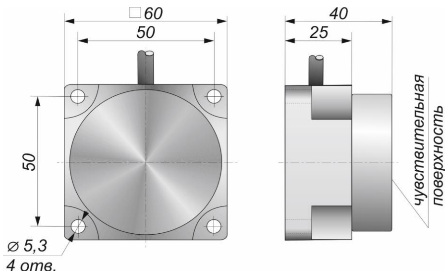
Габаритный чертеж
