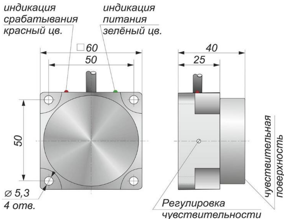
Габаритный чертеж
